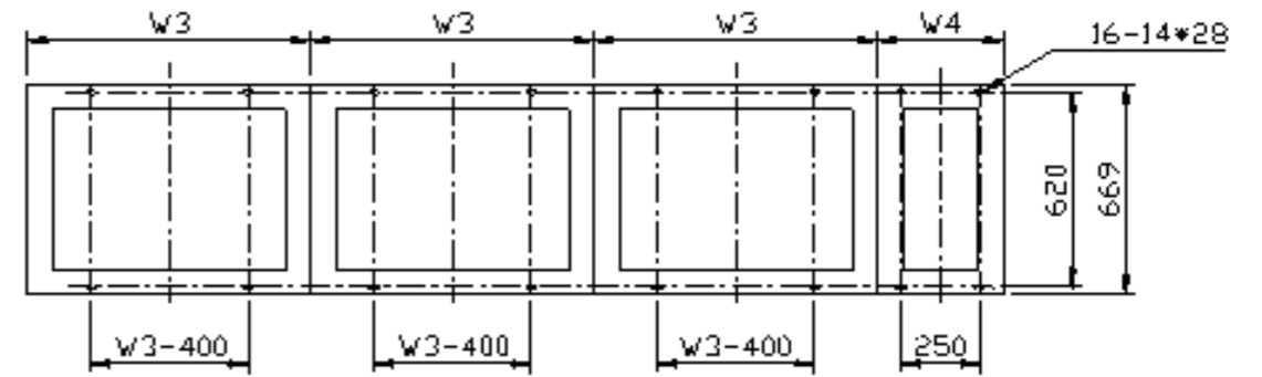
整流回馈HF500A-1500-6-C+P成柜外形示意图
