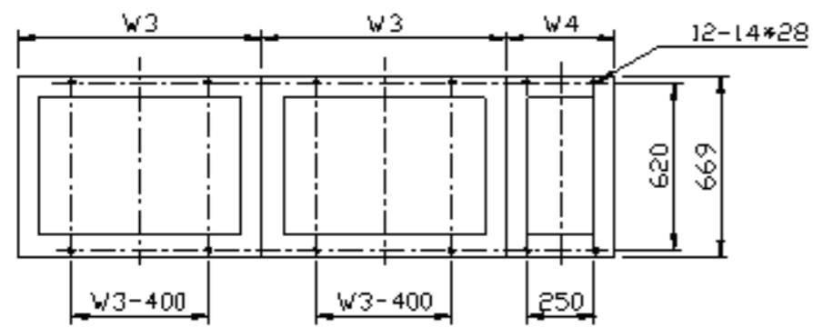
整流回馈HF500A-630-6-C+P、HF500A-800-6-C+P 和HF500A-1000-6-C+P成柜外形示意图
