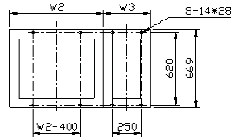
整流回馈HF500A-160-6-C+P、HF500A-250-6-C+P、HF500A-315-6-C+P和HF500A-500-6-C+P成柜外形示意图
